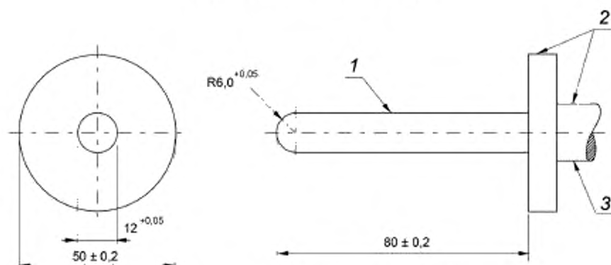
Рисунок 2 — Испытательный штырек
