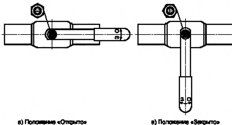
Рисунок 2 — Положение шпнделя и рукоятки в положении «Открыто» и «Закрыто»
