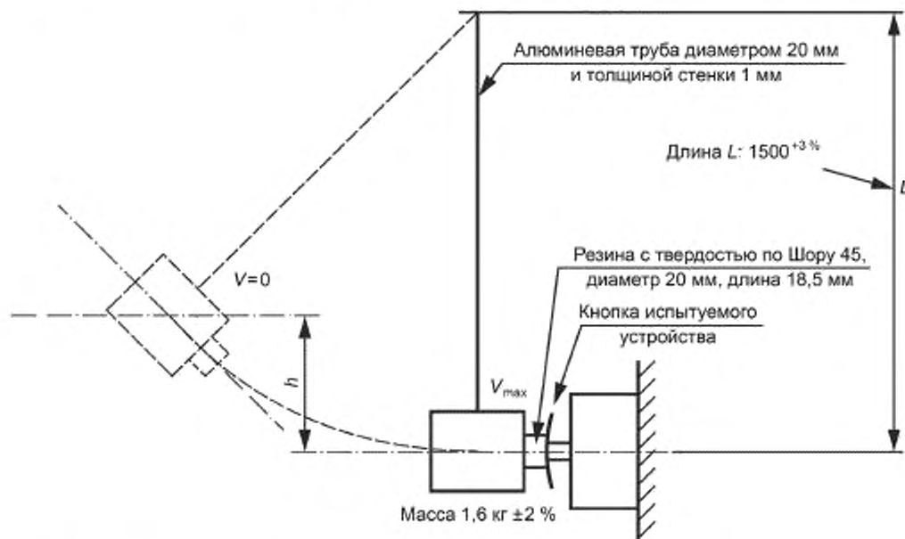
Рисунок 1 — Испытательный боек
