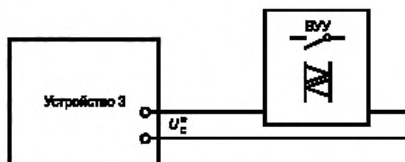
Рисунок G.4 — Контроллеры с единым вводом внутреннего источника питания для цепи управления и вводом для цепи управления
