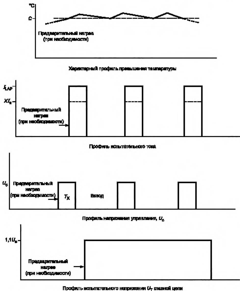
Рисунок F.2 — Профиль испытания на перегрузочную способность
