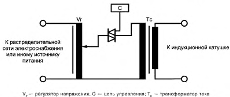
Рисунок 2 — Схема испытательного генератора магнитного поля промышленной частоты
