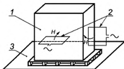
Рисунок 6 — Схема проверки восприимчивости ИО на устойчивость к магнитному полю промышленной частоты методом приближения с использованием индукционной катушки с размером витка 1 × 1 м
