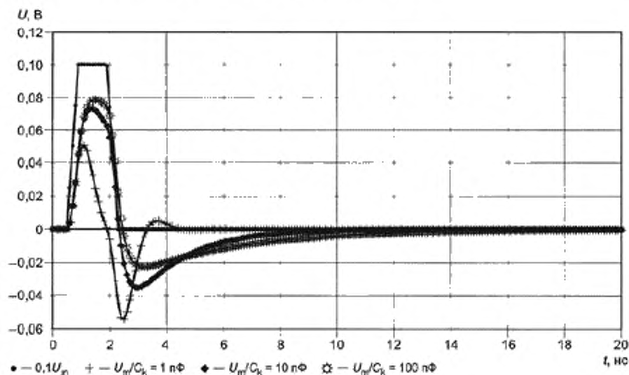
Рисунок D.8 — Входной сигнал U_{in} и измеряемый сигнал U_m , зависящие от емкости конденсатора связи C_k (емкость испытуемого образца C_3 = 10 пФ) [5]
