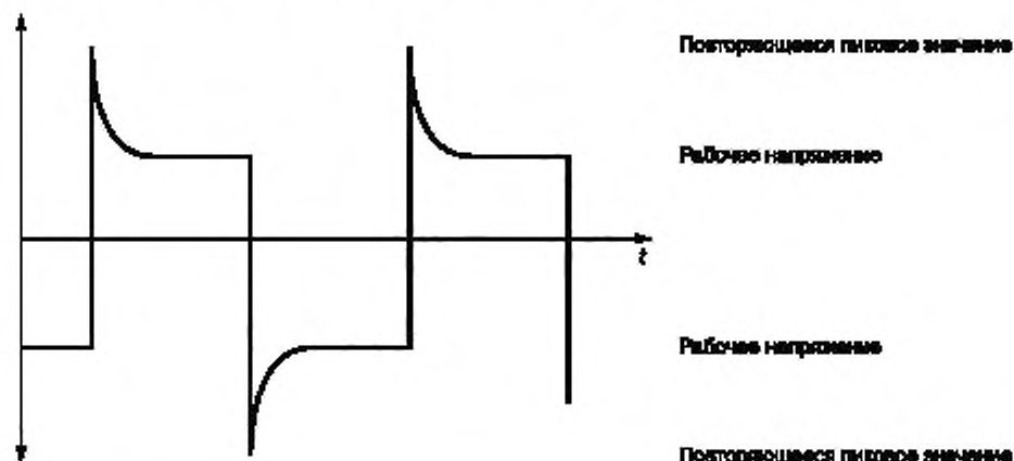
Рисунок 4 — Периодическое импульсное напряжения (см. IEC 60664-1)
