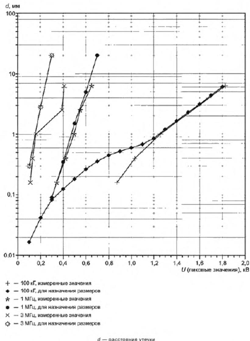
Рисунок 2 — Размеры расстояний утечки, исключая случаи ЧП (расстояния утечки не менее 1 мм) или пробоев (расстояния утечки менее 1 мм)
