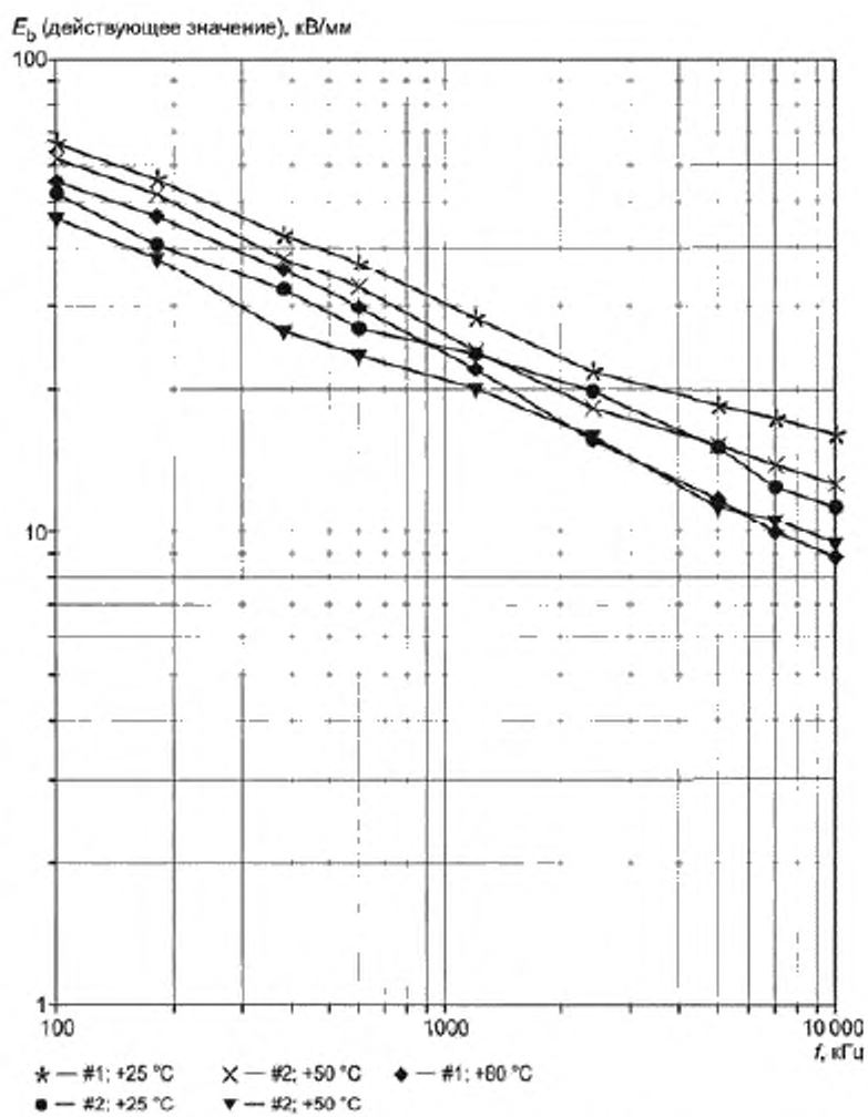
Рисунок С.6 — Высоочастотный пробой изолирующих пленок; #1 — полистирол, d = 80 мкм; #2 — полиэтилен, d = 50 мкм [20]
