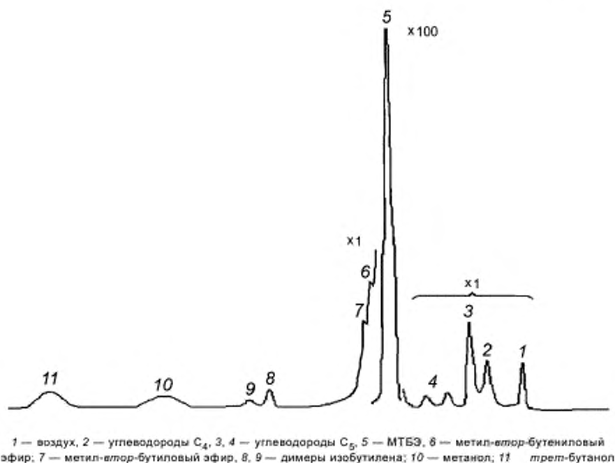
Рисунок 1 — Хроматограмма метил- трет -бутилового эфира на колонке с ТВИН-60
