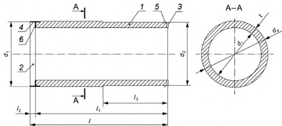
1 — бетонная часть трубы, 2 — раструбная стальная обечайка, 3 — упорное кольцо; 4 — уплотнитель, 5 — уплотнительная манжета; 6 — компрессионное кольцо; d_1 — внутренний диаметр трубы, d_2 — наружный диаметр трубы; t — толщина стенки трубы; l_1 — внутренний диаметр раструбной обечайки; d_2 — диаметр втулочного конца трубы; l, l_1, l_3 — размеры трубы по ее длине; l_2 — глубина раструба
