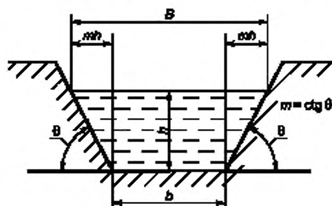
Рисунок 1 — Схема оросительного канала трапецеидального сечения
