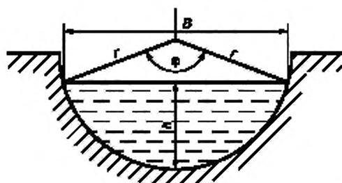
B — ширина поверху; h — глубина воды в канале; r — радиус живого сечения, \varphi — центральный угол сечения
