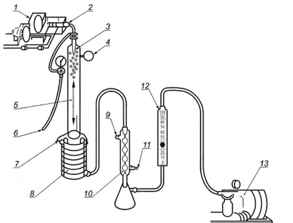
1 — приводной механизм; 2 — взвесь бактерий; 3 — распылитель; 4 — фильтр; 5 — аэрозольная камера, 6 — источник воздуха высокого давления; 7 — тестируемый материал; 8 — микробиологический проботборник; 9 — выход для раковины; 10 — конденсатор, 11 — вход для холодной воды; 12 — откалиброванный расходомер; 13 — компрессор (вакуумный насос)
