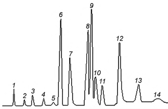
1 — воздух; 2 — пропан; 3 — пропен; 4 — циклопропан; 5 — пропадиен; 6 — изобутан; 7 — n -Бутан; 8 — бутен-1; 9 — изобутен; 10 — транс -Бутен-2; 11 — цис -Бутен-2; 12 — бутадиен-1,3; 13 — изопентан; 14 — n -Пентан
