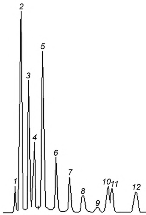
1 — метан; 2 — этан + этилен; 3 — пропан; 4 — пропен; 5 — изобутан; 6 — n -Бутан; 7 — бутен-1 + изобутен; 8 — транс -Бутен-2; 9 — цис -Бутен-2; 10 — изопентан; 11 — бутадиен-1,3; 12 — n -Пентан
