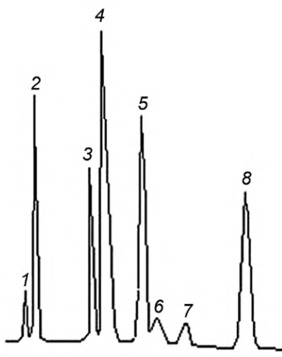
Рисунок Б.6 — Типовая хроматограмма пропан-пропиленовой фракции установки пиролиза на колонке с ТЗК/ВМ
