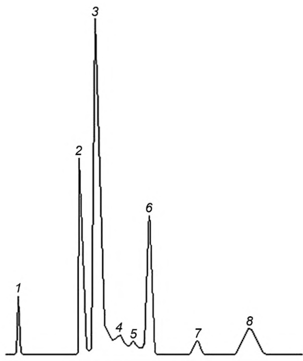
1 — воздух; 2 — изобутан; 3 — n -Бутан; 4 — бутен-1; 5 — изобутен; 6 — транс -Бутен-2 + 2,2-диметилпропан; 7 — цис -Бутен-2; 8 — изопентан
