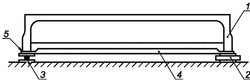
1 — изделие; 2 — шарнирно-неподвижная опора; 3 — каток; 4 — швеллер; 5 — сварной шов
