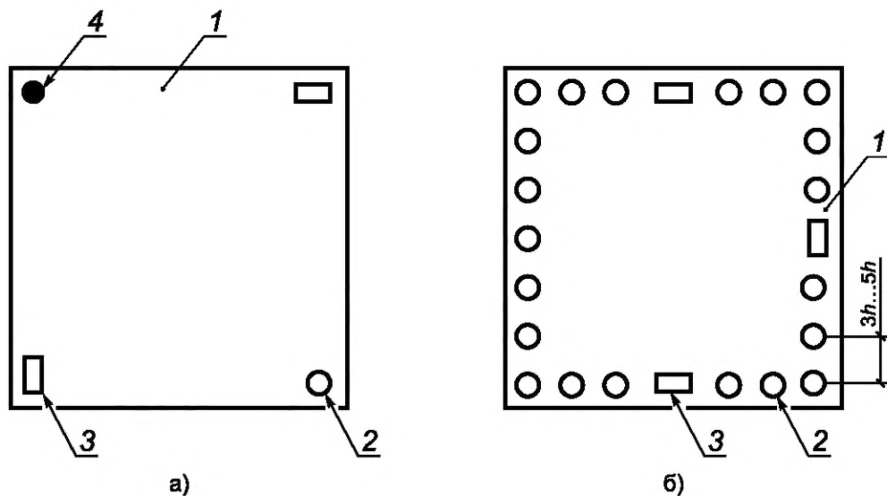
а) Опираие по четырем углам; б) Опираие по четырем сторонам 1 — изделие; 2 — шарнирно-подвижная опора; 3 — каток; 4 — шарнирно-неподвижная опора
