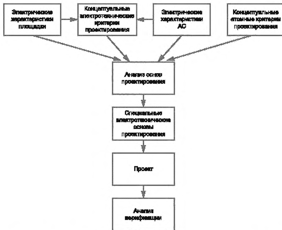
Рисунок А.1 — Входные данные и процесс по определению электротехнических проектных основ для атомных станций, а также анализа верификации
