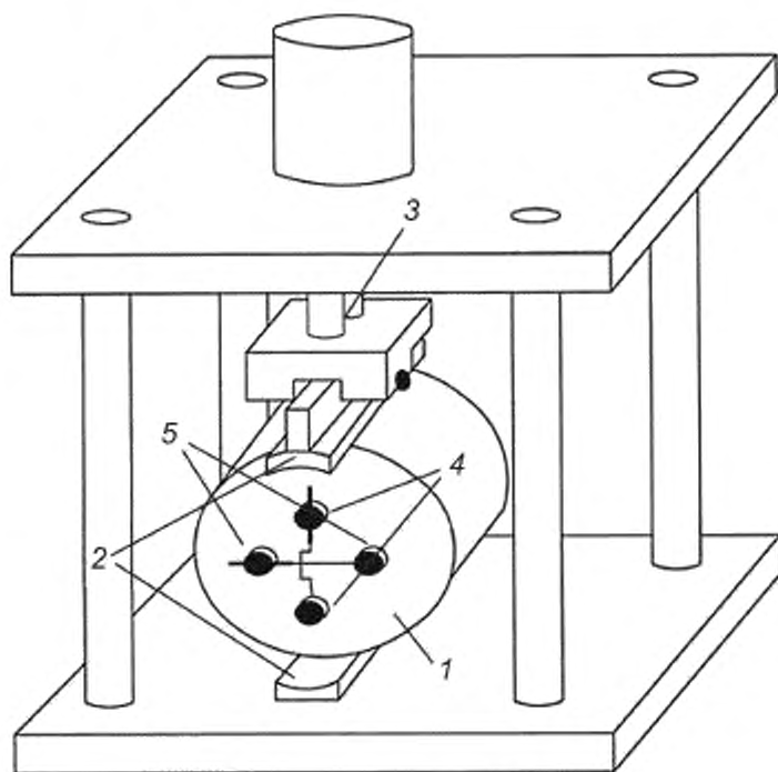
1 — образец асфальтобетона; 2 — нагрузочные пластины; 3 — нагрузочное устройство; 4 — вертикальные датчики перемещений; 5 — горизонтальные датчики перемещений
