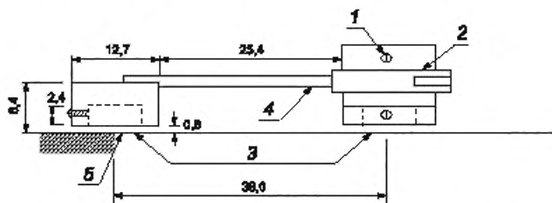
1 — крепежный винт датчика LVDT; 2 — стержень в сборе. 3 — места установки латунных таблеток 4 — латунная трубка наружным диаметром 1,6; 5 — поверхность образца
