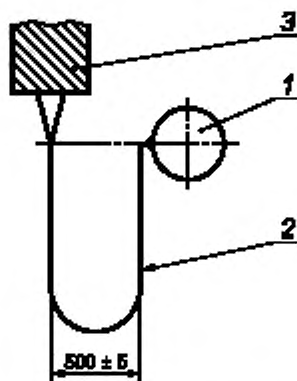
Рисунок 4 — Схема испытаний образца веревки на воздействие динамической нагрузкой
