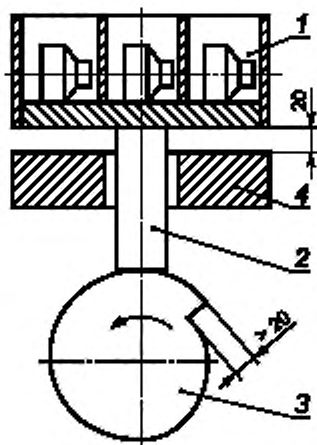
1 — стальная коробка; 2 — поршень; 3 — кулачок; 4 — стальная пластина
