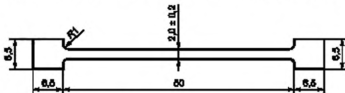
Рисунок 3 — Узкий испытуемый образец
