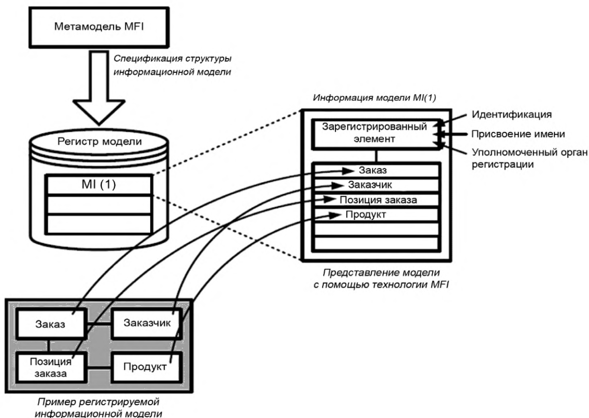
Рисунок 8 — Соотношение между моделью и ассоциированной информацией
