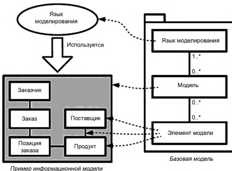
Рисунок 10 — Понятие базовой модели
