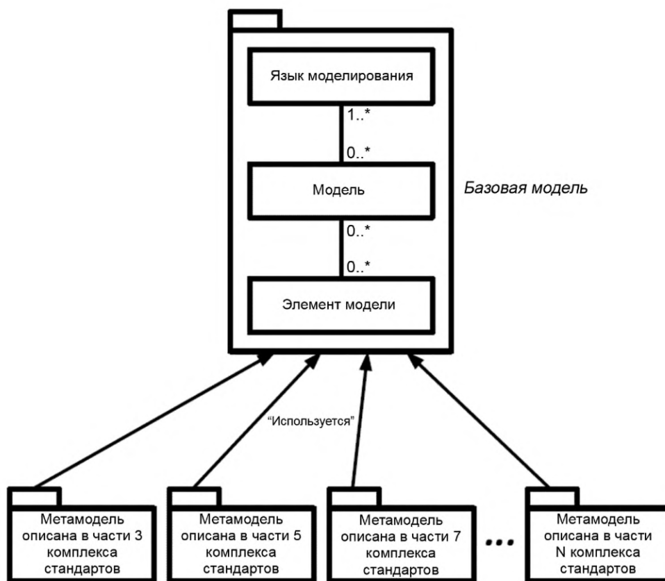
Рисунок 11 — Общая база частей комплекса стандартов MFI
