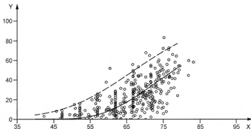
X — оценочный уровень шума на интервале «день — вечер — ночь» L_{den} , дБ; Y — доля населения, испытывающего сильное раздражение от действия шума P_{HA} , %
