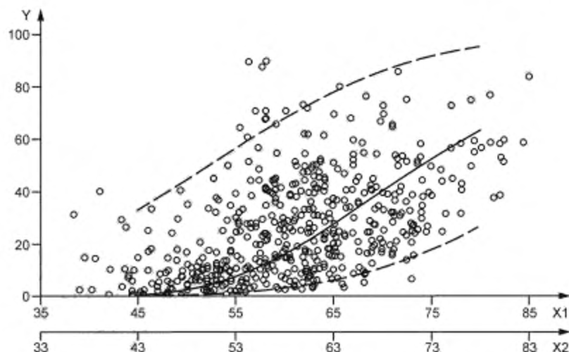
X1 — оценочный уровень шума на интервале «день — вечер — ночь» L_{ден} , дБ, с поправкой 5 дБ; X2 — оценочный уровень шума на интервале «день — вечер — ночь» L_{ден} , дБ, с поправкой 7 дБ; Y — доля населения, испытывающего сильное раздражение от действия шума P_{HA} , %
