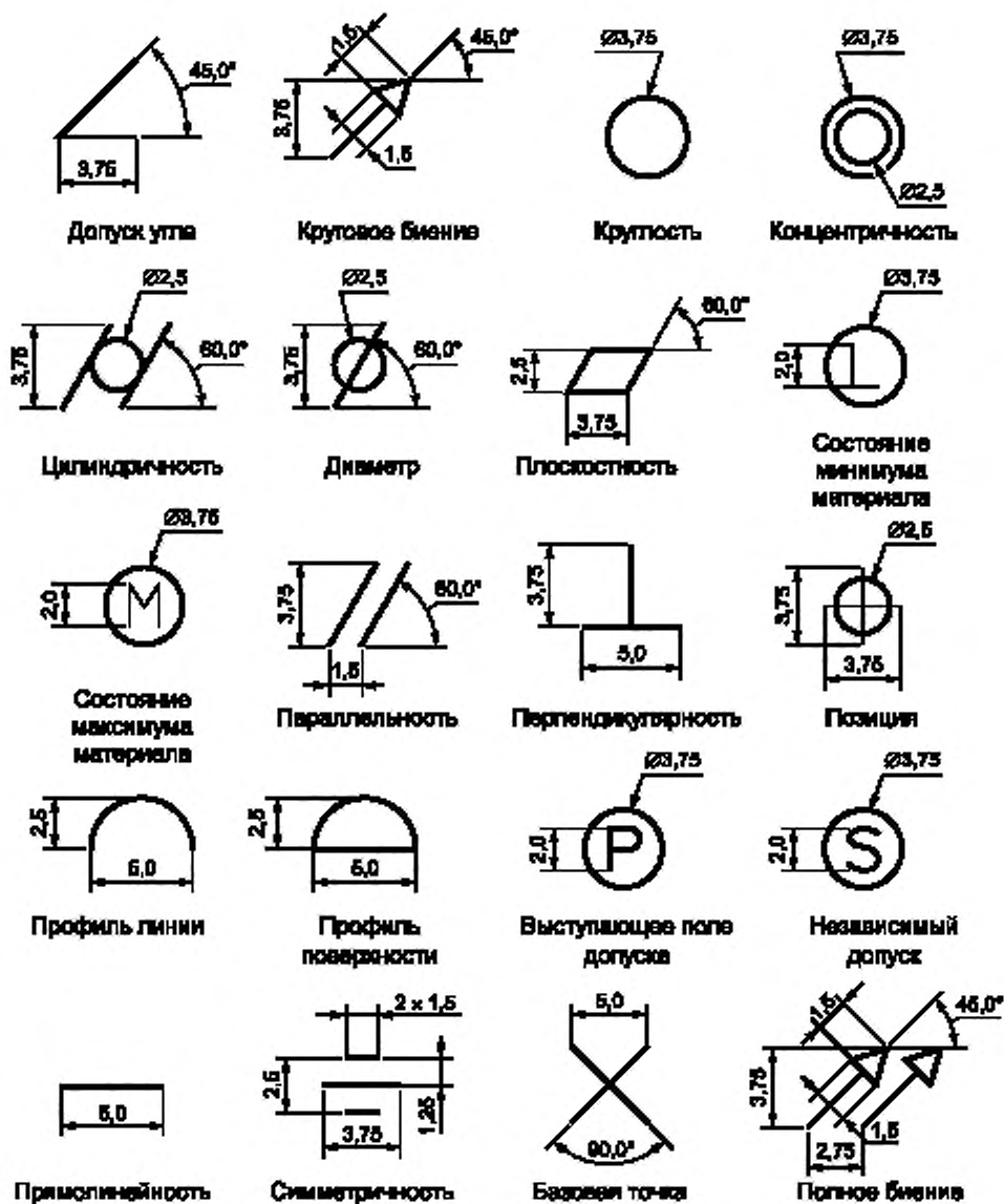
Рисунок 3 — Предопределенные условные обозначения геометрических допусков
