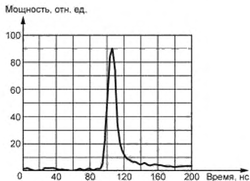
Рисунок А.1 — Форма импульса
