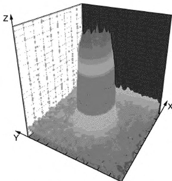
Рисунок А.2 — Профиль пучка
