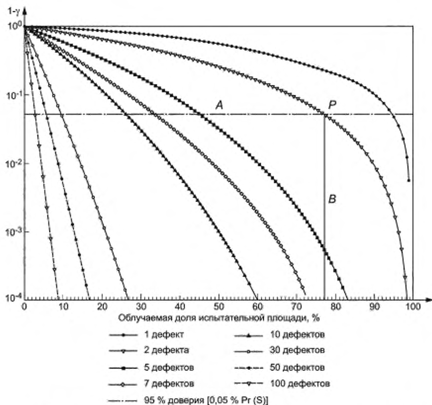
Рисунок В.1 — Облучаемая доля испытательной площади, которую необходимо подвергнуть испытаниям для достижения уровня доверия \gamma , для разных значений N_d
