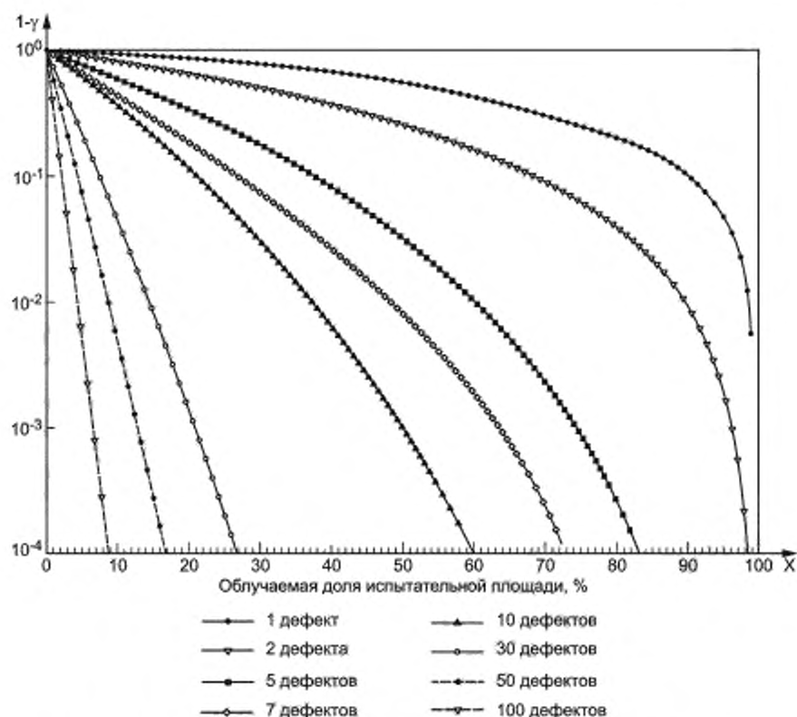
Рисунок С.1 — График операционно-характеристической зависимости
