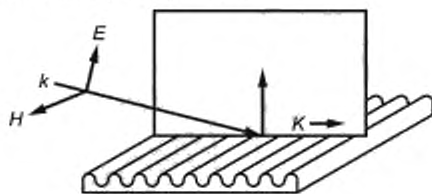
Рисунок 8 — p-поляризация
