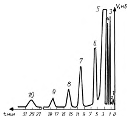
1 — воздух; 2 — винилиденхлорид; 3 — транс -дихлорэтилен; 4 — цис -дихлорэтилен + 1,1,1-трихлорэтан + хлороформ; 5 — трихлорэтилен; 6 — перхлорэтилен + 1,1,2-трихлорэтан; 7 — н -декан; 8 — 1,1,1,2-тетрахлорэтан + 1,1,2,2-тетрахлорэтан; 9 — пентахлорэтан; 10 — гексахлорэтан
