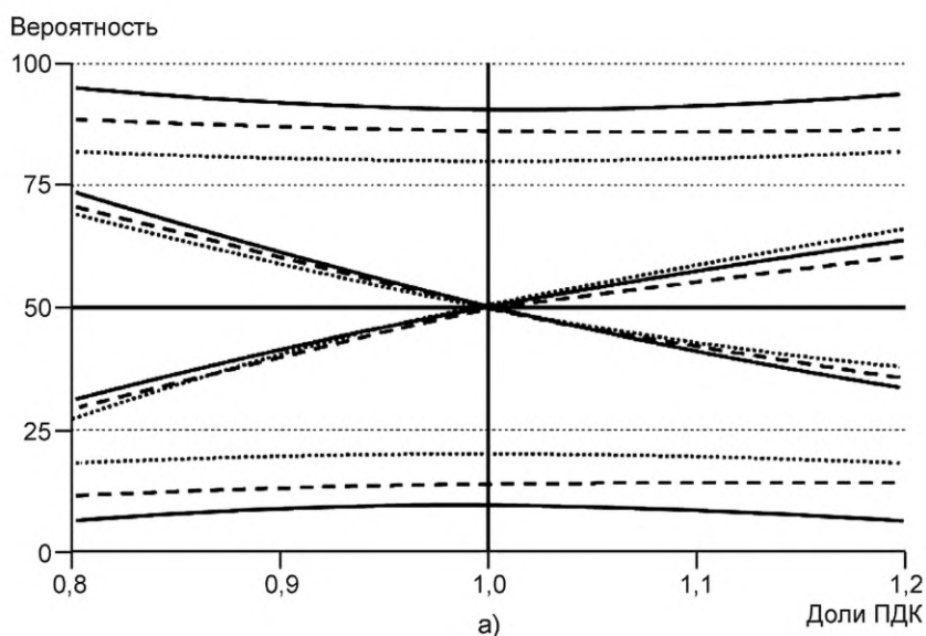
Рисунок 1 — Зависимость вероятности, %, принятия правильных и ложных решений о соответствии/несоответствии качества воды установленным требованиям от концентрации загрязняющего вещества, выраженной в долях ПДК 2) , при следующих равенствах:
