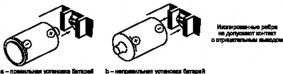
Рисунок В.2 — Положительный контакт, утопленный между ребрами
