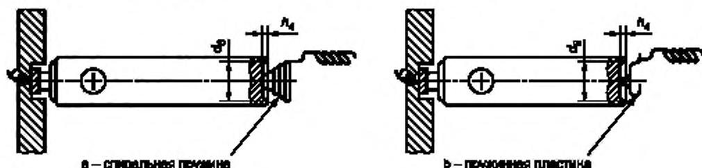
Рисунок В.12 — Примеры отрицательных контактов
