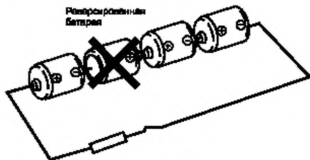
Рисунок В.1 — Пример последовательного соединения с одной реверсивированной батареей
