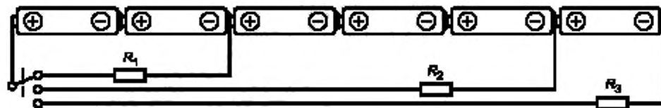
Рисунок В.13 — Пример дробного отведения напряжения при последовательном соединении батареи
