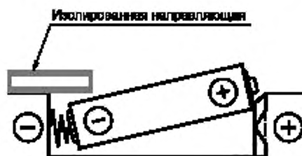
Рисунок В.11 — Один из примеров защищенной установки
