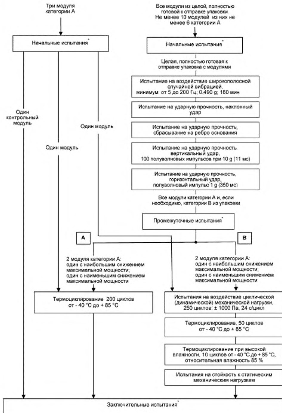
Рисунок 1 — Порядок проведения испытаний фотоэлектрических модулей
