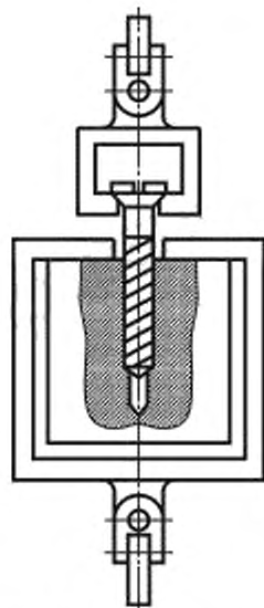
Рисунок 2 — Схема выдергивания шурупа из кромки плиты
