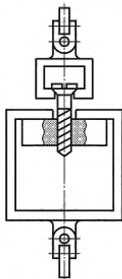
Рисунок 1 — Схема выдергивания шурупа из пласти плиты
