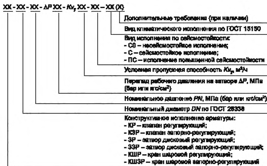
Рисунок 1 — Схема условного обозначения арматуры
