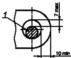
Рисунок 8 — Установка задвижки с проушинами под навесной замок
