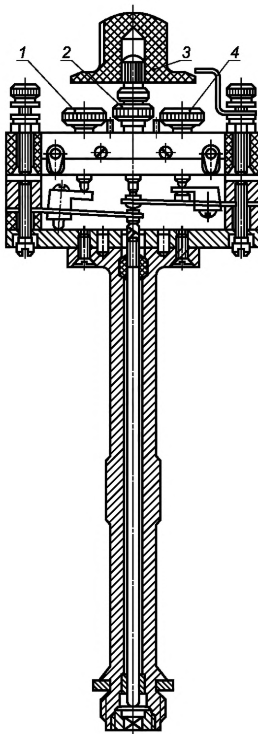
Рисунок 4 — Продольный разрез индикатора воспламенения
