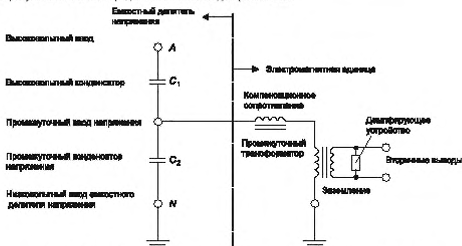
Рисунок 5A.1 — Пример диаграммы для емкостного трансформатора напряжения
