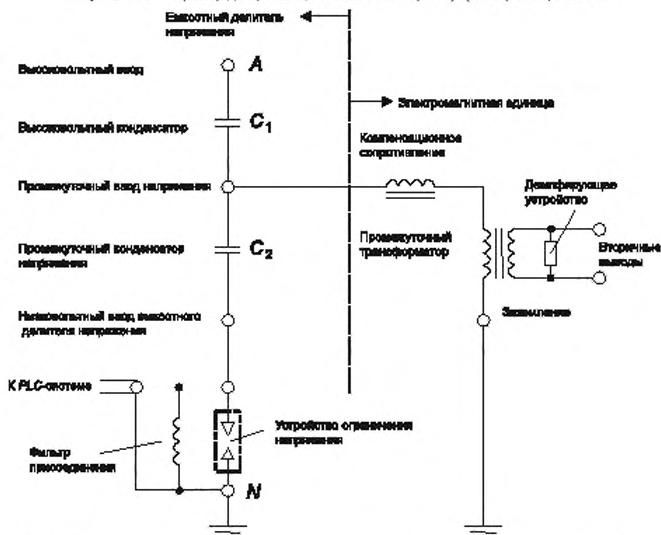
Рисунок 5A.2 — Пример диаграммы для емкостного трансформатора напряжения с вспомогательным частотным оборудованием
