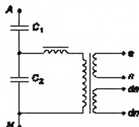
Рисунок 505 — ETC с одной обмоткой напряжения нулевой последовательности и одной вторичной обмоткой
