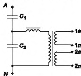
Рисунок 503 — ETC с двумя вторичными обмотками
