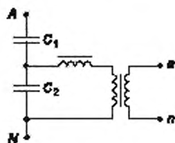
Рисунок 502 — ETC с одной вторичной обмоткой
