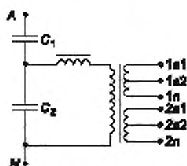
Рисунок 504 — ETC с двумя секционированными вторичными обмотками
