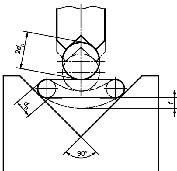
Рисунок 1 — Прогиб f
