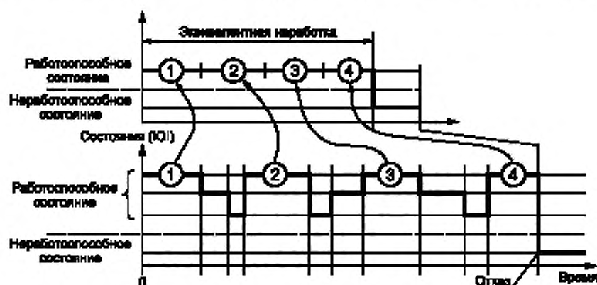
Рисунок 13 — Эквивалентная наработка для объектов IOI
