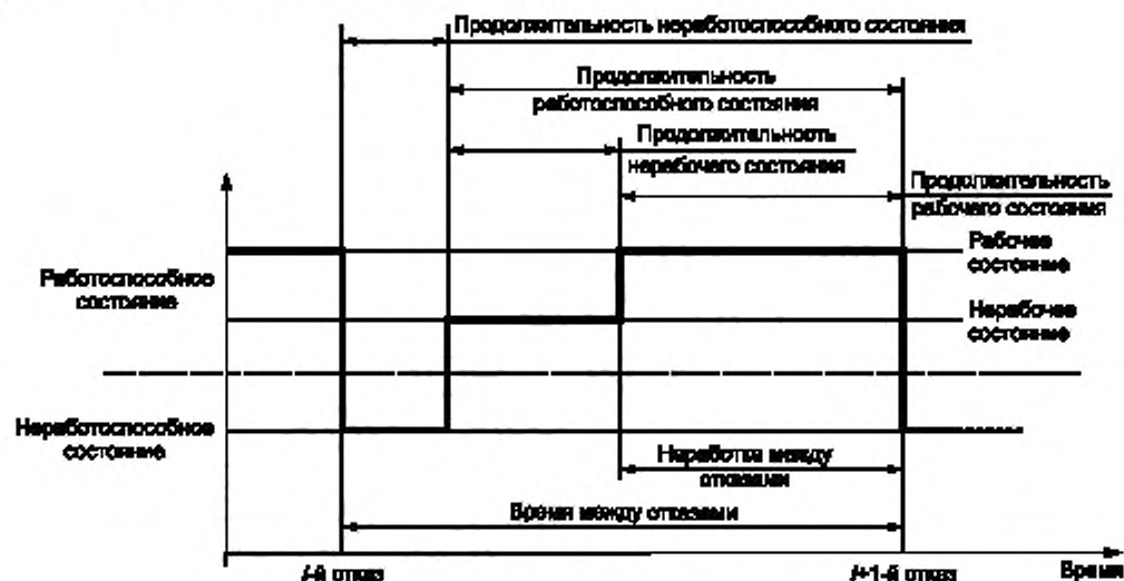
Рисунок 28 — Время между отказами и наработка между отказами
