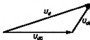
Рисунок 3 — Иллюстрация вектора эмиссии U_{d1} и его вклада в измеряемый вектор помех U_d от установки в РОЕ
