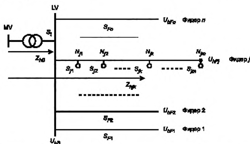
Рисунок D.4 — Упрощение общей схемы общественной низковольтной системы для расчета уровней гармонических напряжений в дальнейшей точке фидеров низковольтных систем
