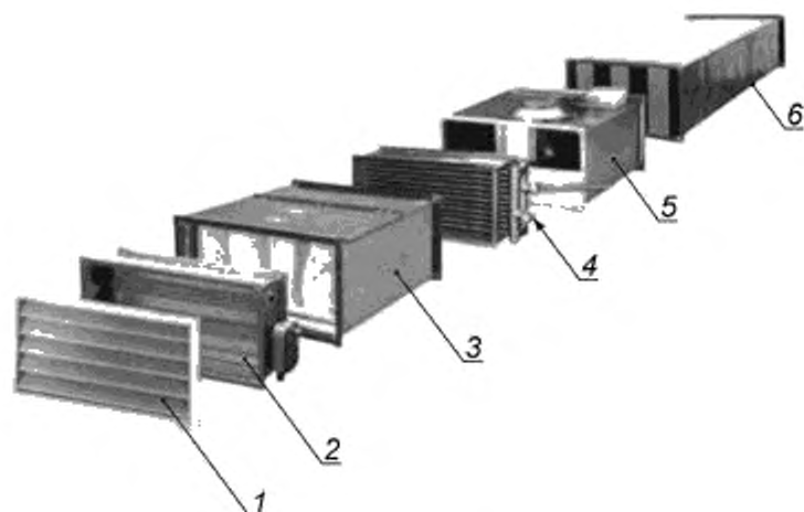
1 — уличная решетка; 2 — клапан с электроприводом; 3 — фильтр; 4 — водяной нагреватель; 5 — каналный вентилятор; 6 — шумоглушитель
