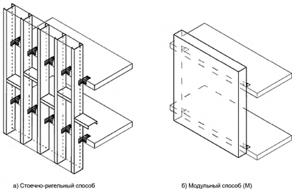
Рисунок 10 — Классификация наружных КОС по принципу монтажа
