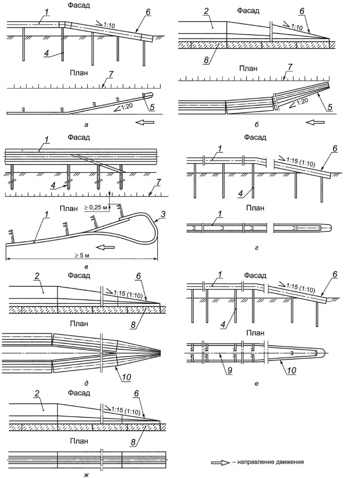
1 — барьерное ограждение; 2 — парапетное ограждение; 3 — изгиб балки ограждения; 4 — стойка ограждения; 5 — отгон ограждения; 6 — понижение ограждения на начальном и конечном участках; 7 — бровка земляного полотна; 8 — основание; 9 — ось разделительной полосы; 10 — сближение рядов ограждения с осью разделительной полосы
