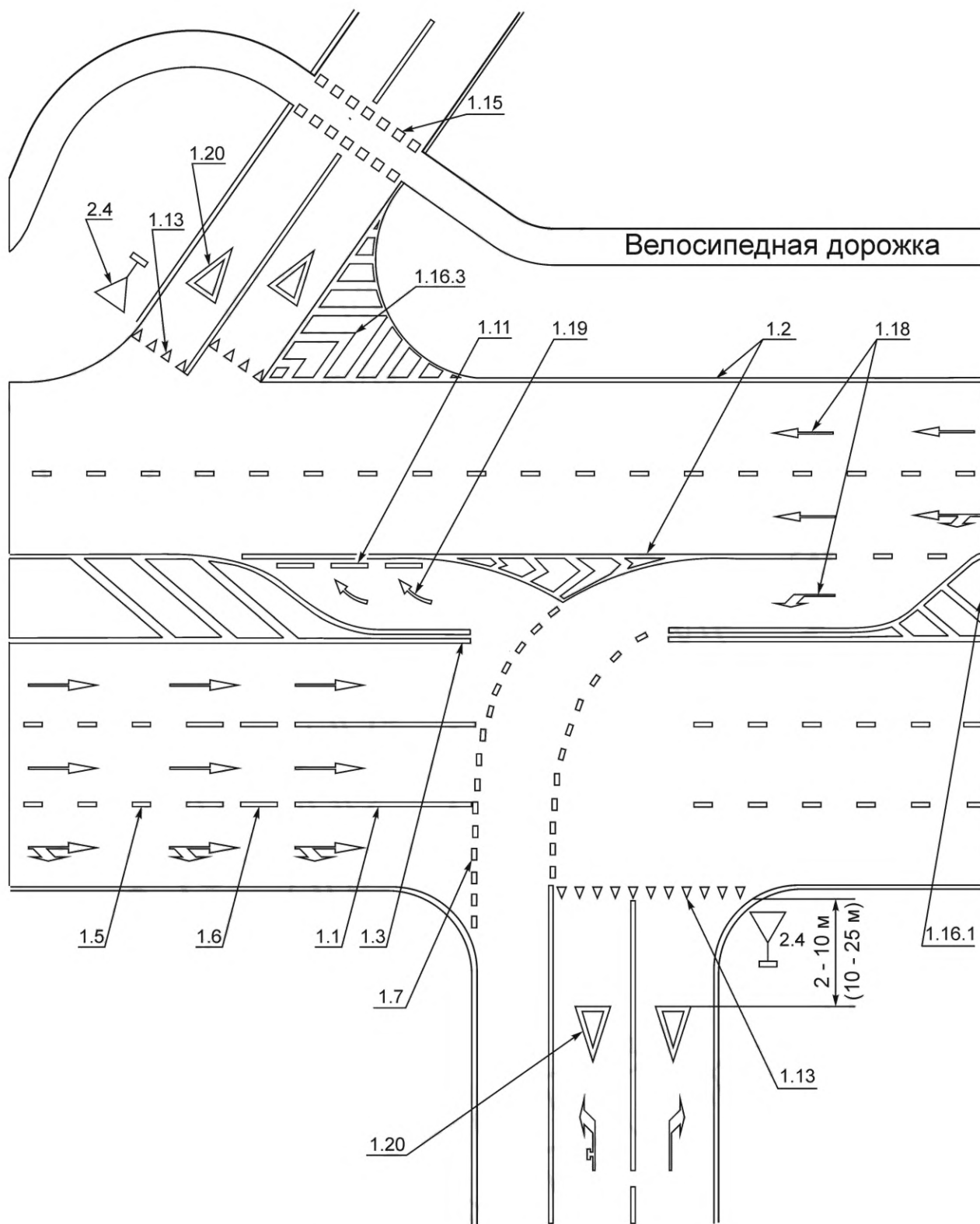
Рисунок В.10 — Пример нанесения разметки канализованного пересечения
