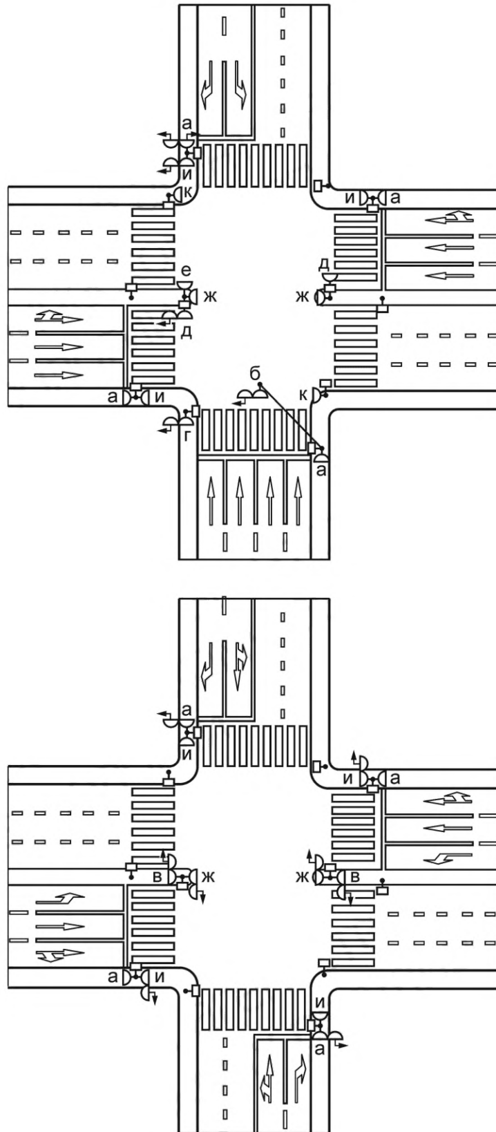
Рисунок В.26 — Места установки светофоров
