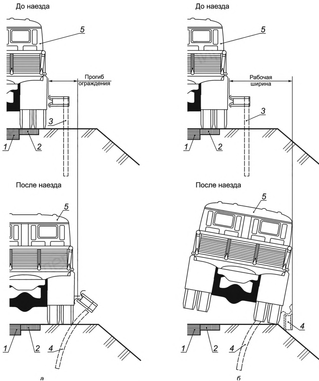
a — прогиб; б — рабочая ширина дорожного ограждения 1 — проезжая часть; 2 — укрепительная полоса; 3 — недеформированное ограждение; 4 — деформированное ограждение; 5 — транспортное средство
