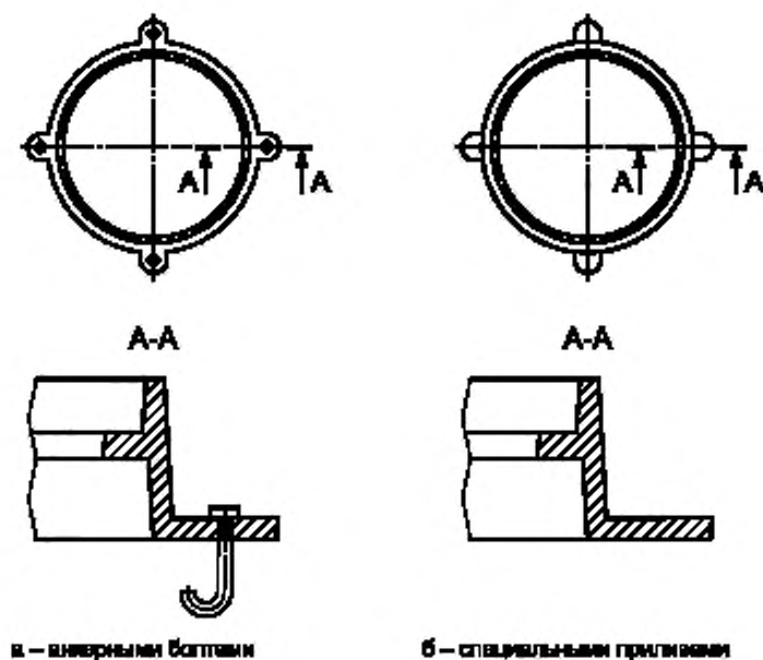
Рисунок А.4 — Усиленная заделка корпуса
