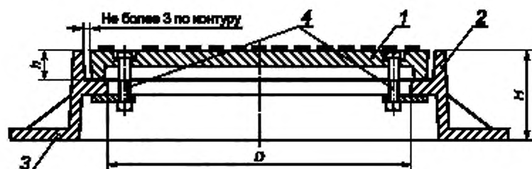
Рисунок А.1 — Люк общего назначения
