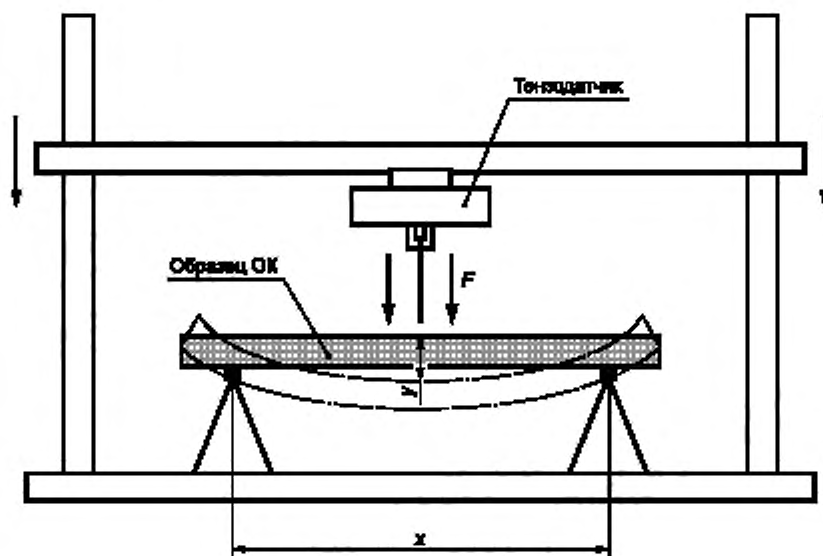
Рисунок 19 — Метод E17A. Схема проведения испытания
