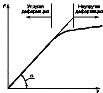
Рисунок 20 — Пример результатов приложения нагрузки и перемещения
