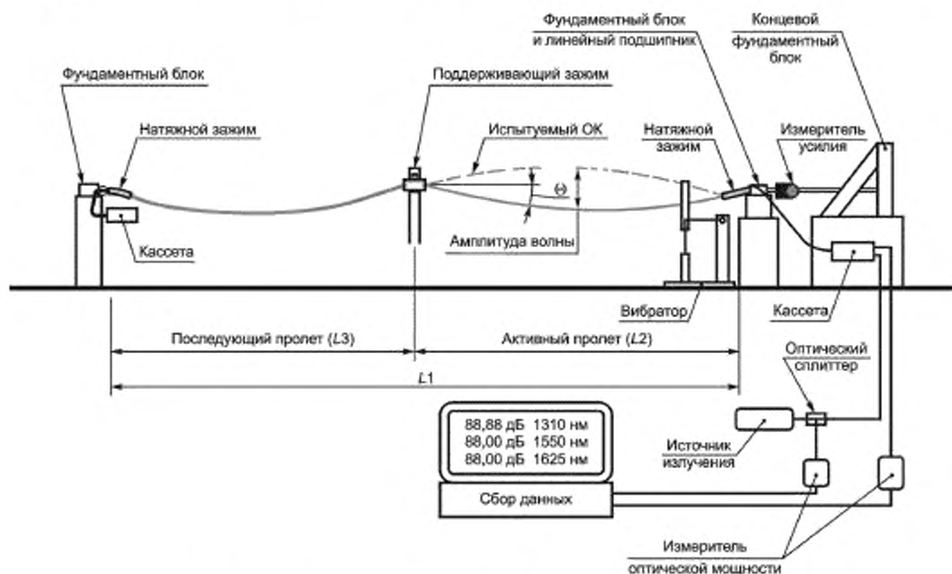
Рисунок 33 — Схема испытания ОК на галоирование (пьяска ОК)
