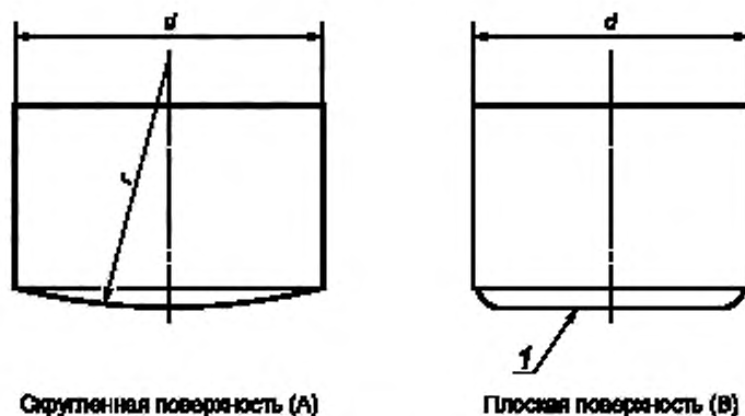
d — диаметр бойка, (20 \pm 1) мм; r — радиус скругления ударной поверхности, 300 мм мин; 1 — плоская ударная поверхность со скругленными кромками s — Испытание на удар. Ударная поверхность бойка
