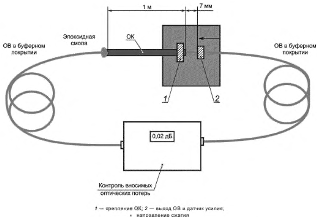
Рисунок 31 — Схема испытания ОВ на перемещение при сжатии
