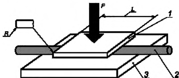
R — радиус кромки подвижной плиты, 5 мм; F — усилие, прикладываемое к подвижной плите; L — длина плиты, 100 мм. 1 — перемещаемая плита; 2 — испытуемый ОК; 3 — неподвижная плита
