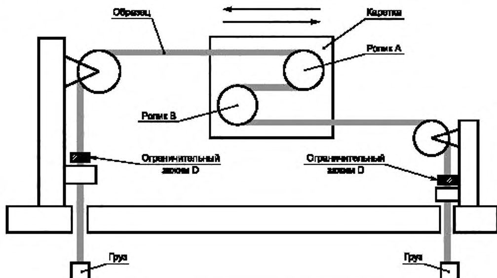
Рисунок 12 — Схема оборудования для испытания на изгиб
