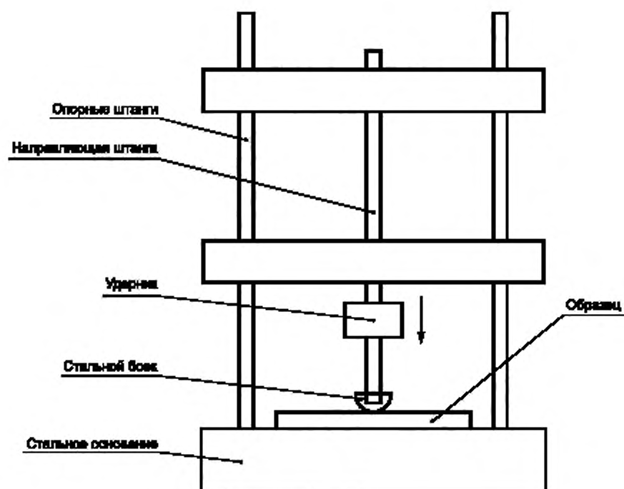
а — Испытание на удар. Схема стэнда для испытаний на воздействие одиночных ударов
