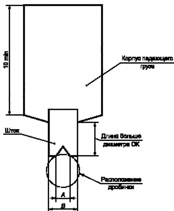
Рисунок 16 — Схема падающего груза, в который встроен шток крепления дробинки
