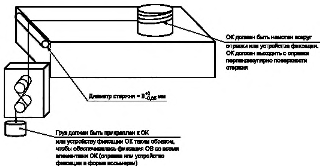
Рисунок 35 — Схема устройства для испытания на механическую надежность
