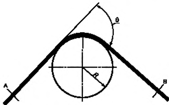
Рисунок 25 — Схема частичного изгиба
