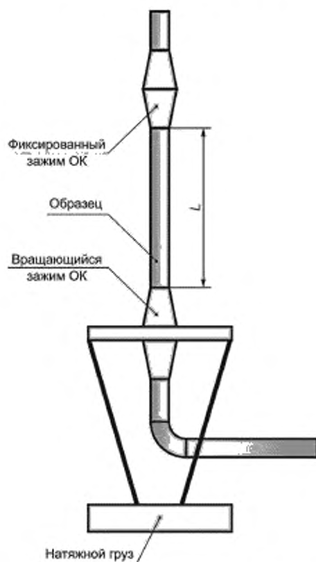
Рисунок 11 — Схема альтернативного оборудования осевого кручения ОК, содержащего натяжной груз
