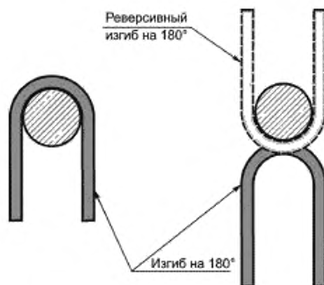
Рисунок 14 — Схема оснастки для испытания на изгиб
