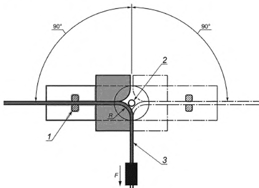
1 — зажим; 2 — ось вращения; 3 — образец; R — радиус изгиба. F — натяжной груз, если он необходим
