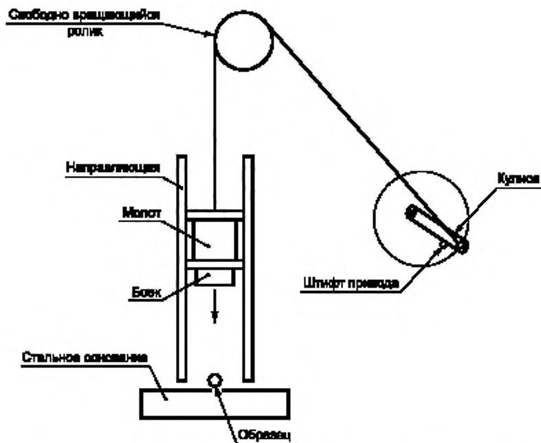
b — Испытание на удар. Схема стенда для испытаний на воздействие многократных ударов
