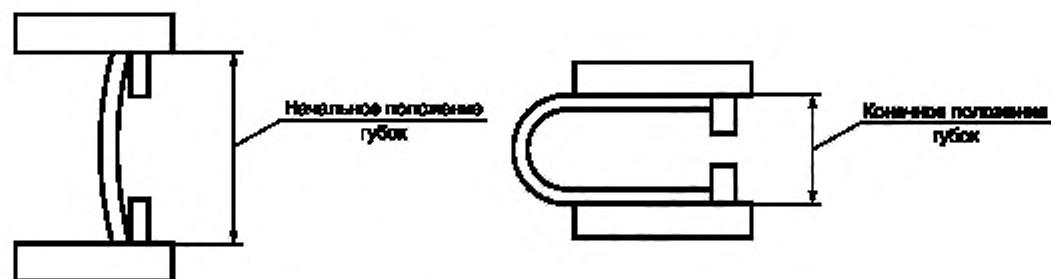
Рисунок 22 — Метод E17C. Схема проведения испытания
