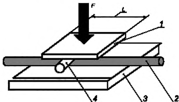
F — усилие, прикладываемое к подвижной плите; L — длина плиты, 100 мм; 1 — перемещаемая плита; 2 — испытуемый ОК; 3 — неподвижная плита; 4 — оправка (цилиндр или полуцилиндр) диаметром 25 мм
