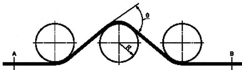
Рисунок 26 — Схема частичного изгиба с использованием нескольких роликов
