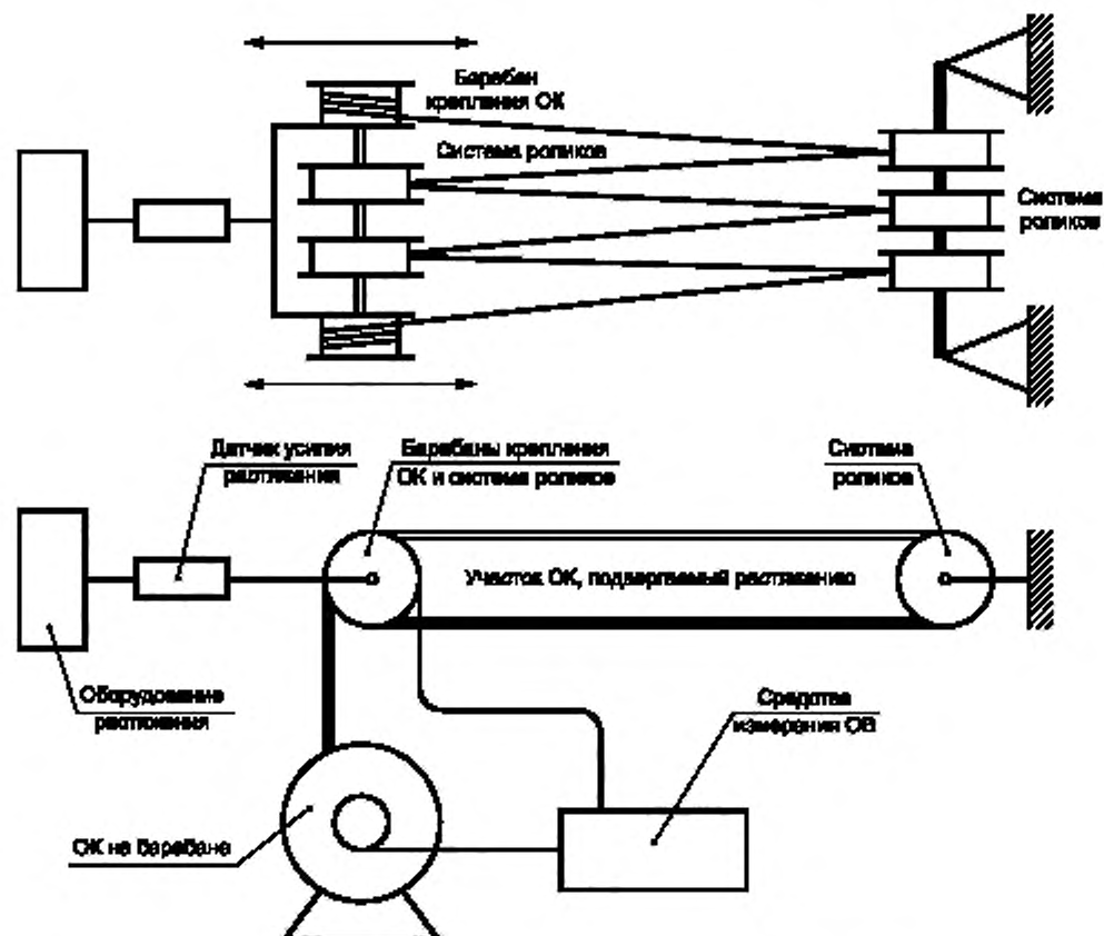
Рисунок 2 — Пример схемы стэнда для испытания ОК на растяжение с использованием систем роликов и барабанов крепления ОК
