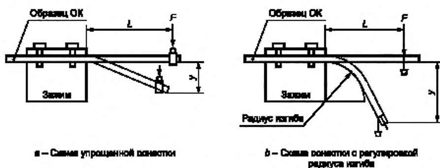
Рисунок 21 — Метод E17B. Схема проведения испытания
