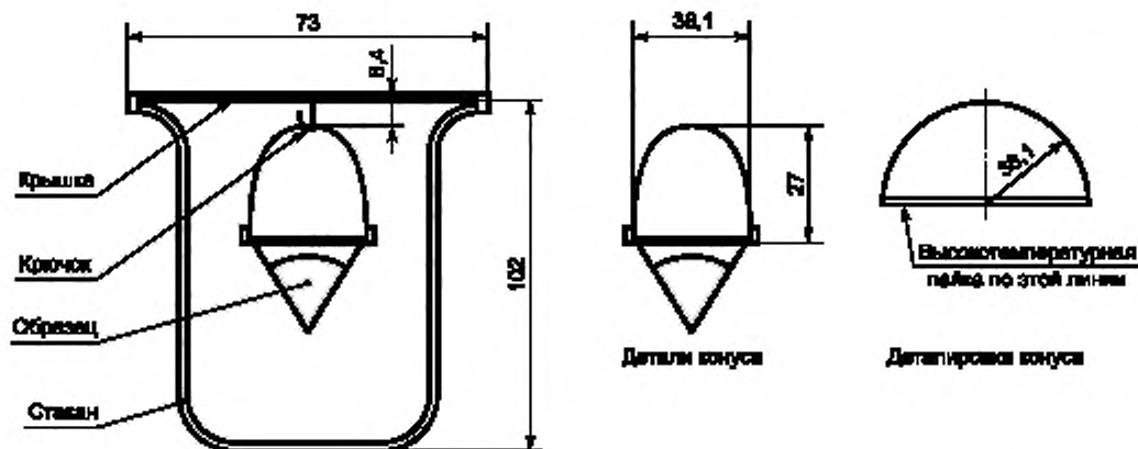
Рисунок 18 — Оснастка для испытания на стекаемость и испарение
