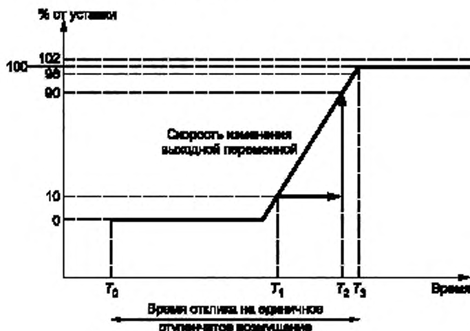
Рисунок 5 — Время отклика на единичное ступенчатое возмущение и скорость изменения выходной переменной СНЭЭ
