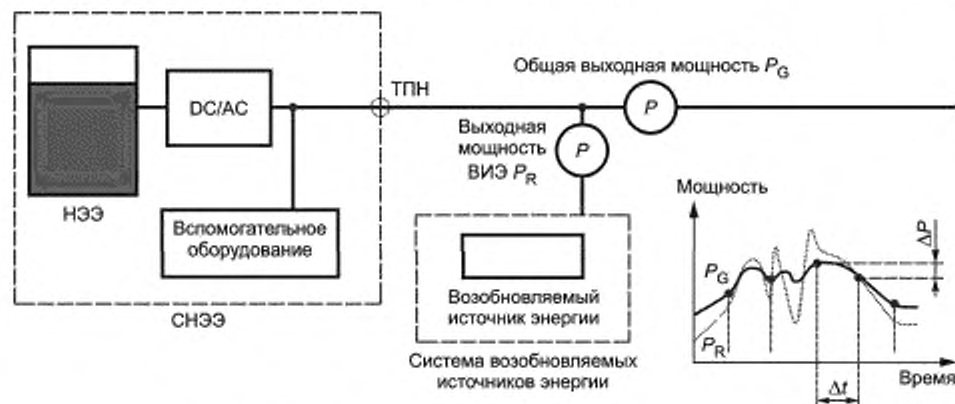
Рисунок В.1 — Испытание на компенсацию колебаний мощности
