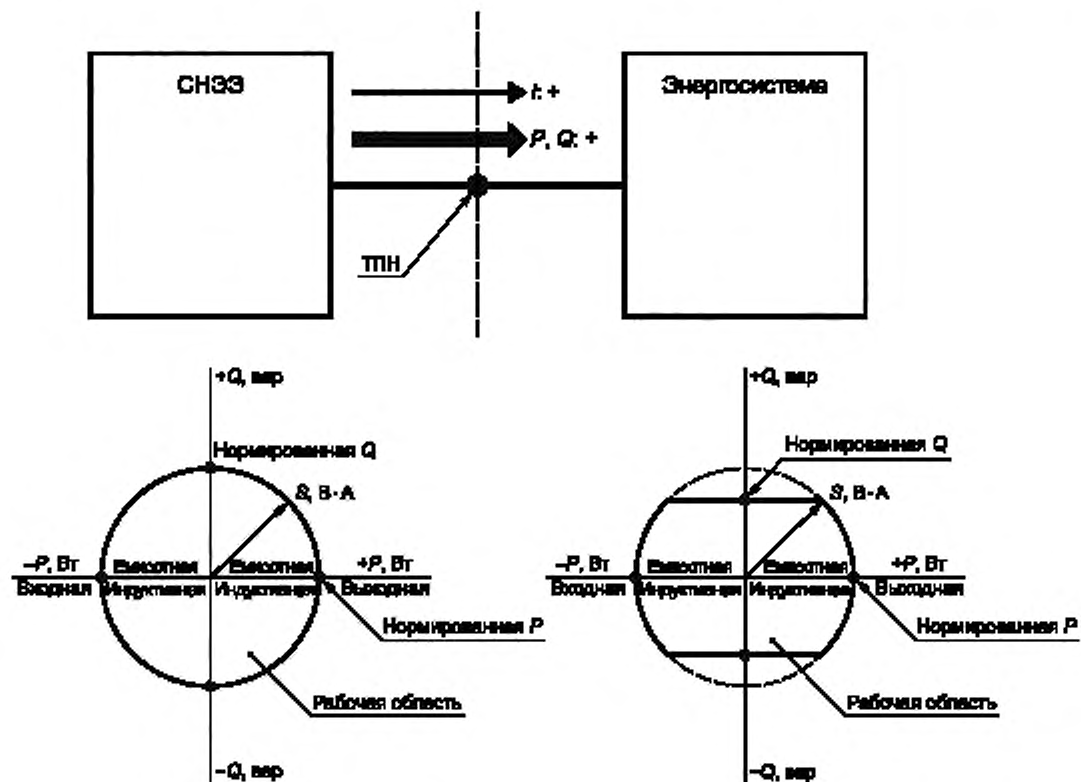
Рисунок 4 — Правило определения направления потоков активной и реактивной мощностей
