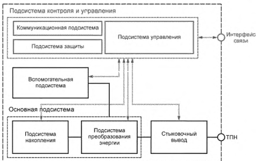
Рисунок 2 — Типовая архитектура СНЭЭ
