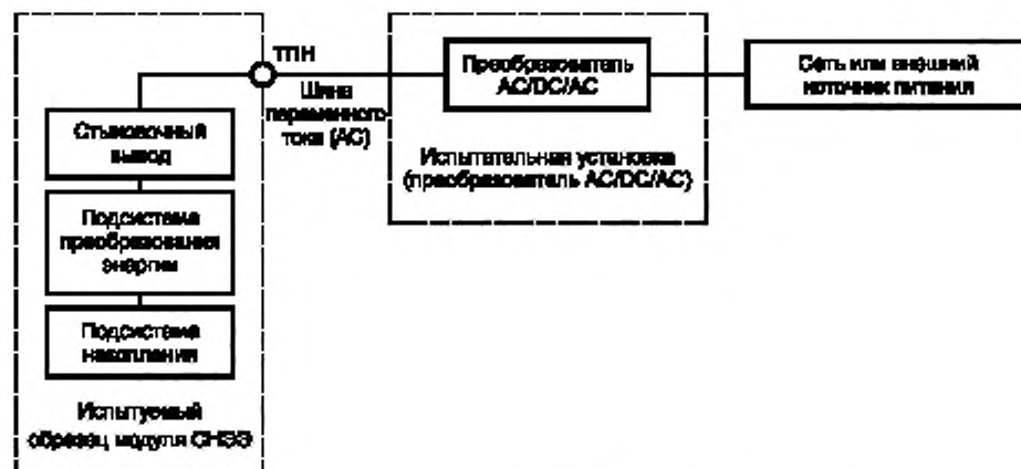
Рисунок С.2 — Схема проведения испытания методом взаимной нагрузки (с преобразователем AC/DC/AC в качестве испытательной установки)
