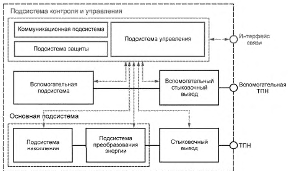
Рисунок 3 — Типовая архитектура СНЭЭ со вспомогательной ТПН
