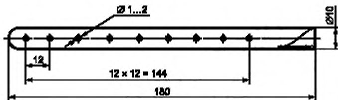
Рисунок 6 — Пробоотборник
