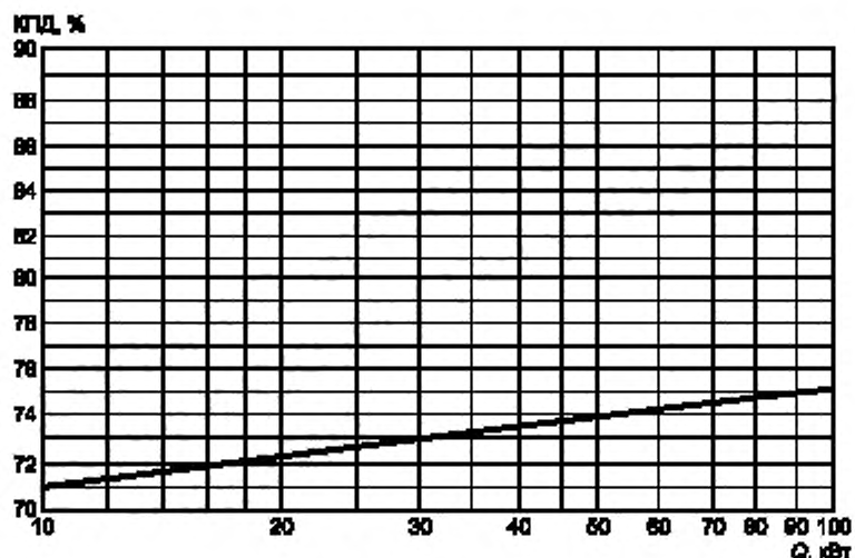
Рисунок 5 — График зависимости КПД котлов для сжигания каменного и бурого углей с выходом летучих веществ от 17 % до 50 % от теплопроизводительности
