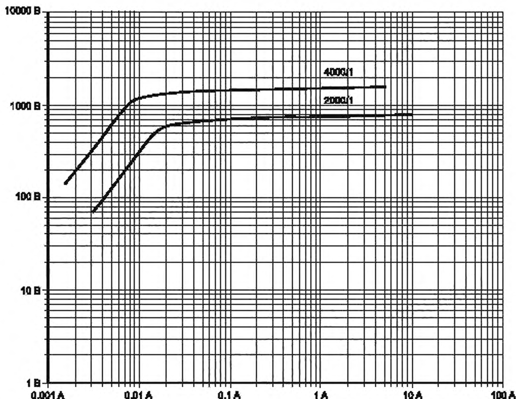
Рисунок В.5 — Вольтамперная характеристика ТТ ЖК ELK СВ3—780 с n_{\text{ном}} 4000/1 (верхняя кривая) и 2000/1 (нижняя кривая)
