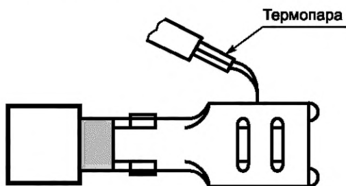
Рисунок К.1 — Пример расположения термодатчика при измерении превышения температуры
