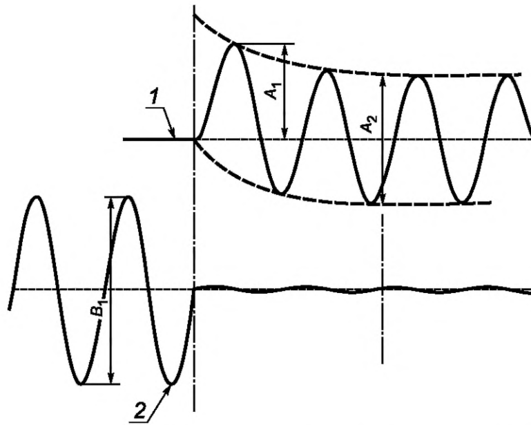
Рисунок 30 — Пример результата калибровки испытания на короткое замыкание [9.11.2.1, перечисление j), 2)]
