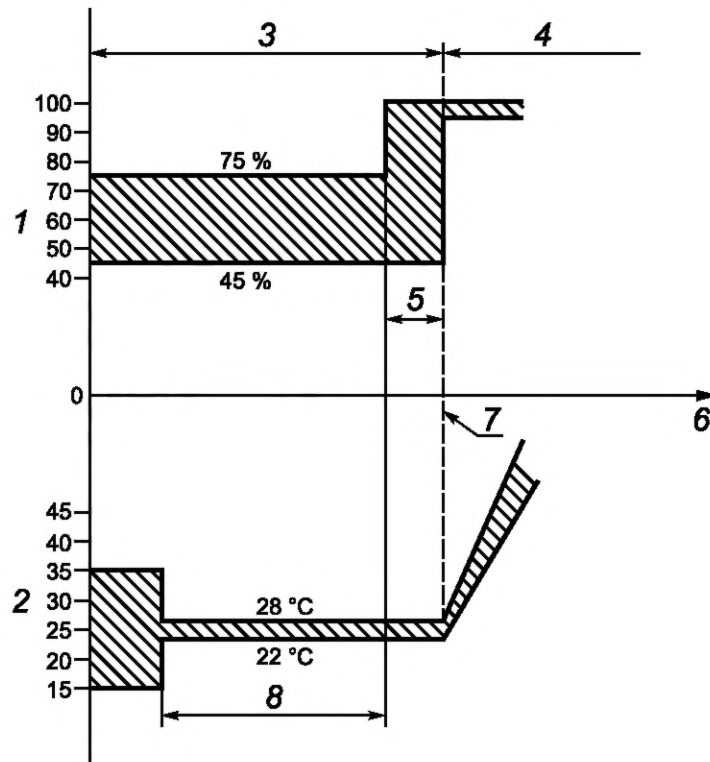
1 — относительная влажность, %; 2 — температура окружающего воздуха, °С; 3 — период стабилизации; 4 — первый цикл; 5 — время, требуемое для достижения 95 % — 100 % относительной влажности (не превышающее 1 ч); 6 — время; 7 — начало первого цикла; 8 — время, требуемое испытываемому образцу, чтобы достичь температурной стабильности
