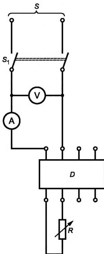
S — источник питания; S_1 — двухполюсный выключатель; V — вольтметр; A — амперметр; D — испытуемый ВДТ; R — переменный резистор
