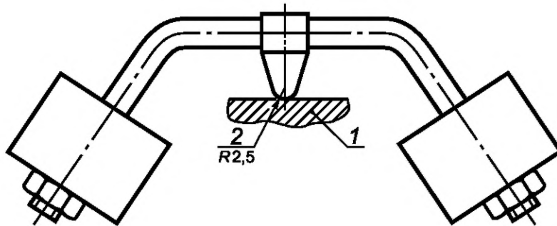
1 — образец; 2 — сфера диаметром 5 мм
