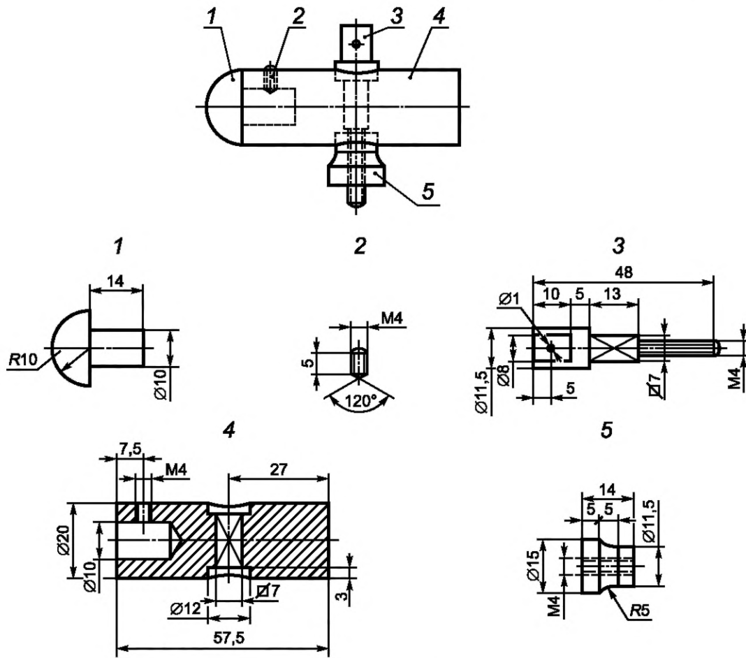
Рисунок 16 — Ударный элемент для маятнкового аппарата для испытаний на механический удар (9.12.2.1)
