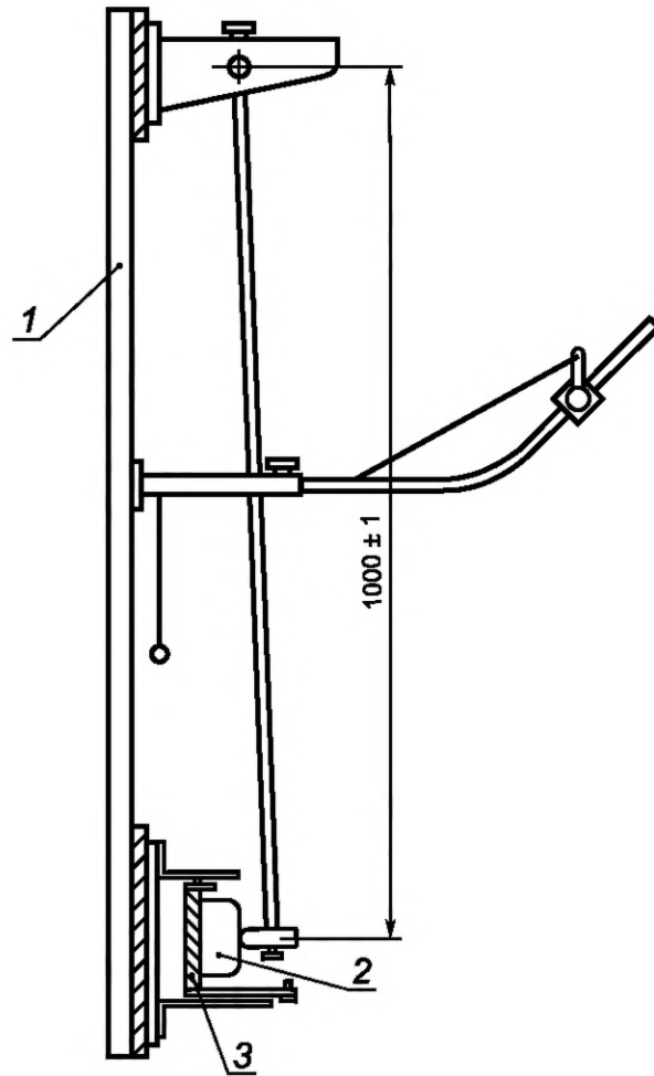
Рисунок 15 — Аппарат для испытаний на механический удар (9.12.2.1)
