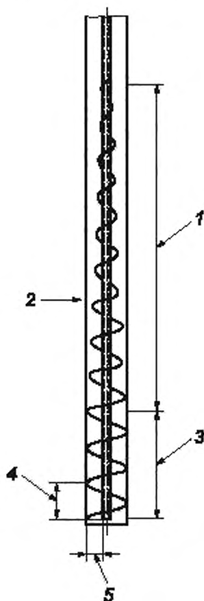
1 — суженные на конус витки; 2 — трубка шнекобура, 3 — полные витки; 4 — шаг витка — три номинальных размера, 5 — кольцевой зазор — три номинальных размера
