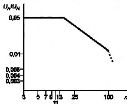
Рисунок 2 — Максимально допустимая гармоническая составляющая номинального напряжения сети
