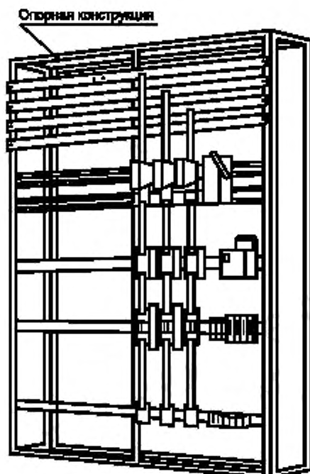
Рисунок С.1 — НКУ заводского изготовления открытого типа
