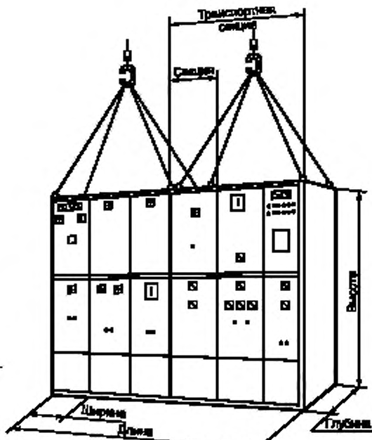
Рисунок С.4 — НКУ заводского изготовления много-шкафного типа
