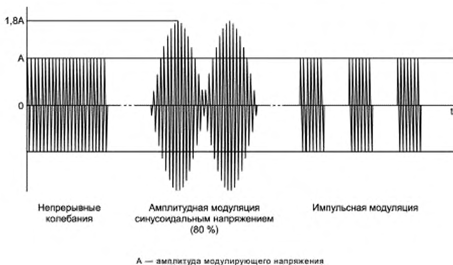
Рисунок 3 — Виды модуляции
