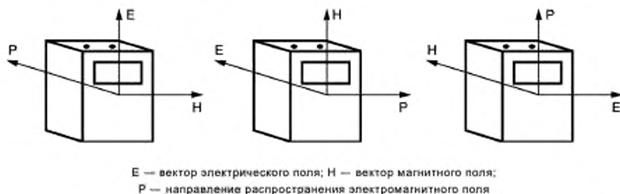
Рисунок 2 — Примеры относительной ориентации ИТС и векторов электромагнитного поля при испытаниях на помехоустойчивость
