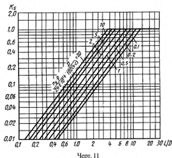
График для определения коэффициента K_5
