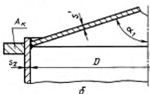
Пологие конические днища
