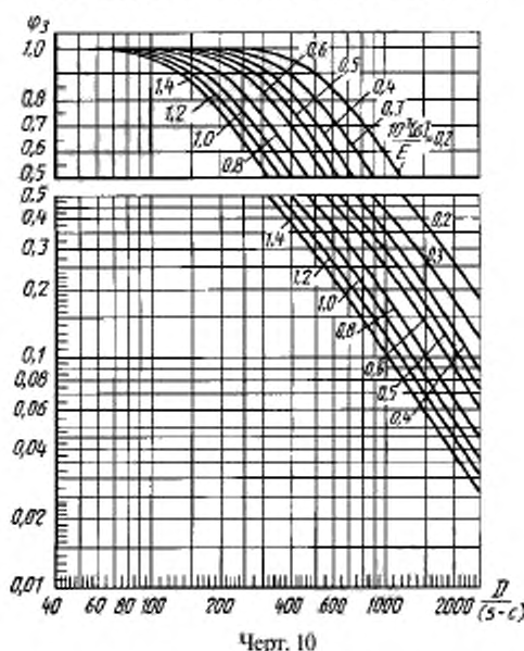
График для определения коэффициента \varphi_3
