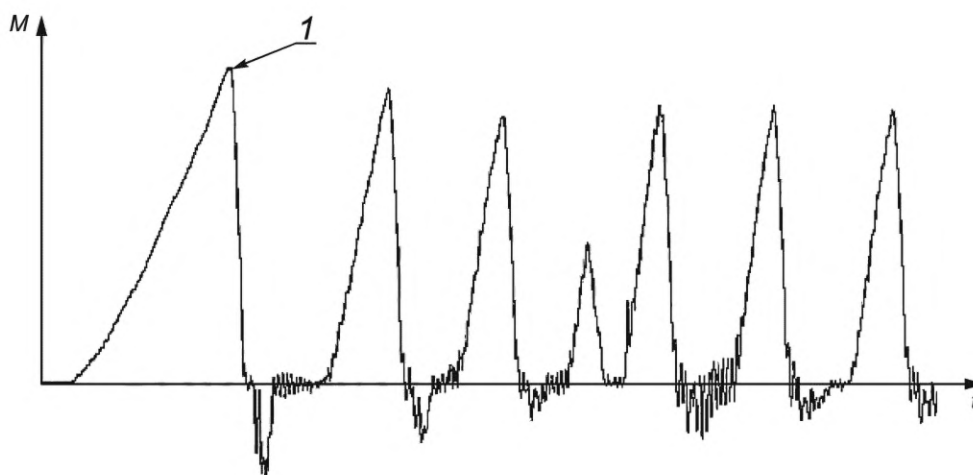
1 — максимальный крутящий момент; M — крутящий момент; t — время
