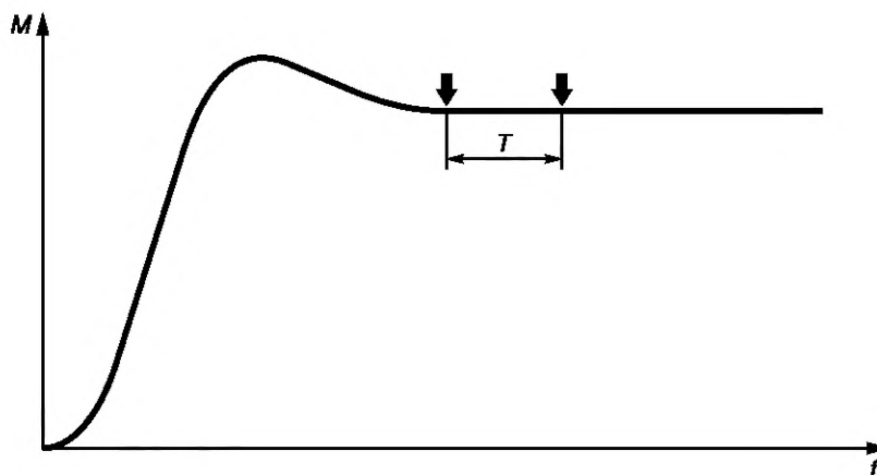
M — крутящий момент; t — время; T — область стабильного сигнала, 2 \text{ мс} < T < 100 \text{ мс}
