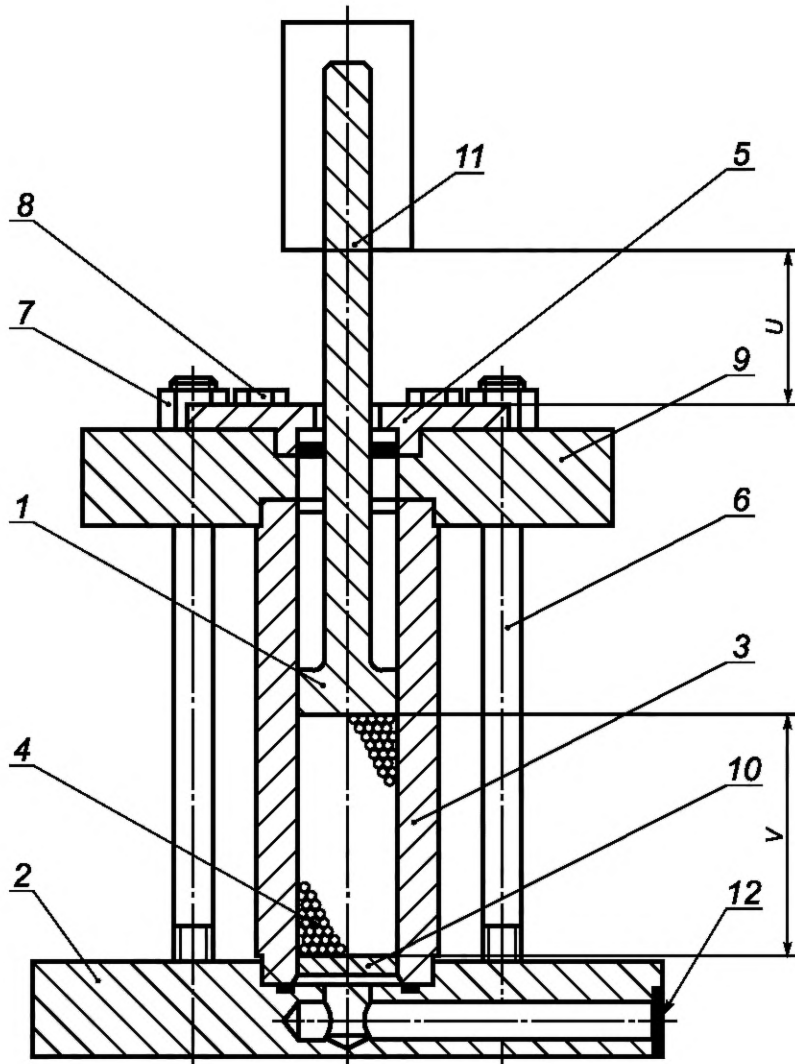
1 — штамп; 2 — нижняя плита; 3 — цилиндр; 4 — закаленные стальные шарики (минимум 63 HRC); 5 — крышка плиты; 6 — резьбовой стержень M16 × 320; 7 — шестигранная гайка M16; 8 — винт с цилиндрической головкой M10 × 25; 9 — фланец; 10 — реакционная тарелка; 11 — хвостовик штампа (для прилегания к патрону инструмента); 12 — вакуумное соединение; V — высота шаровой колонны, см. таблицу AA.1; U — свободная длина штампа (максимум 50 мм)
