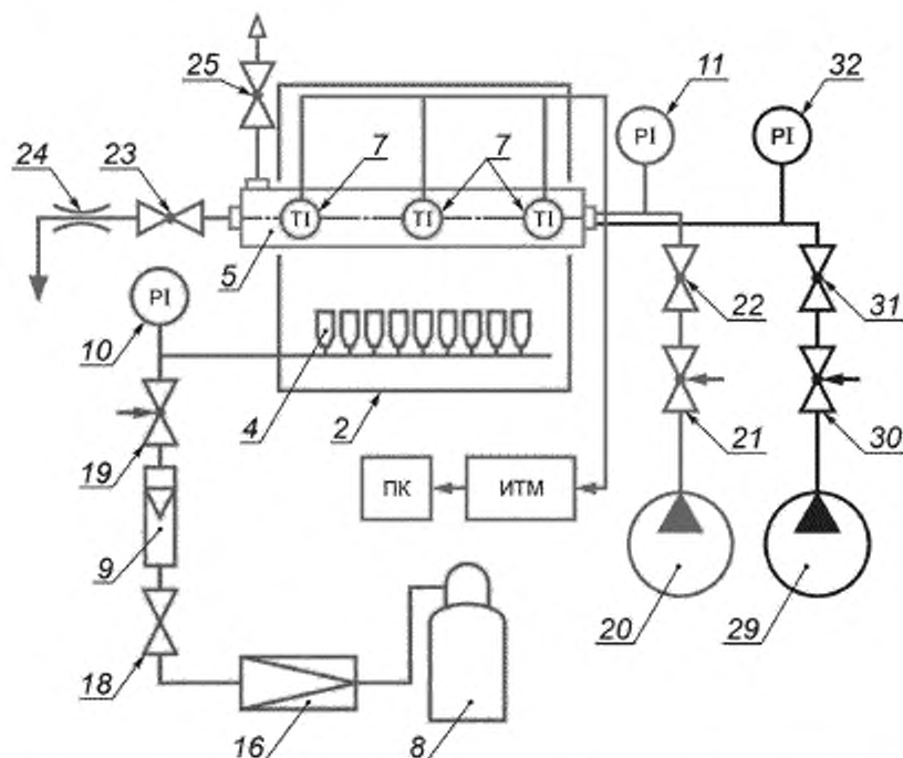
2 - испытательная камера; 4 - газовые горелки; 5 - трубопроводная сборка; 7 - термолары (ТТ); 8 - газовый баллон; 9 - расходомер; 10, 11, 32 - манометры (PI); 16 - редуктор; 18, 22, 23, 25, 31 - краны; 19, 21, 30 - регулирующие устройства; 20 - источник гидравлического давления, 24 - диафрагма; 29 - источник пневматического давления; ПК - персональный компьютер, ИТМ - многоканальный технологический измеритель
