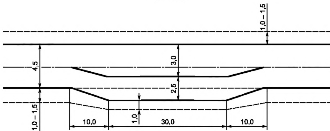
б) Карман
