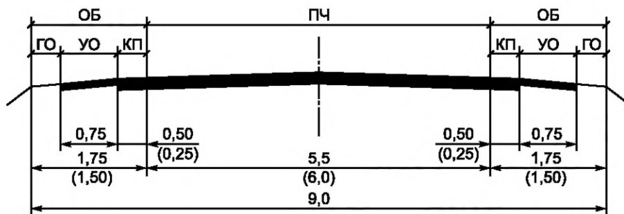
б) Типовой поперечный профиль автомобильных дорог категорий IVБ-р
