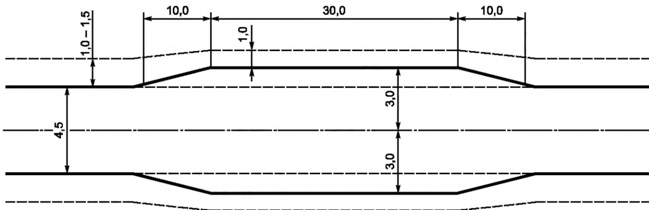
а) Разъезд
